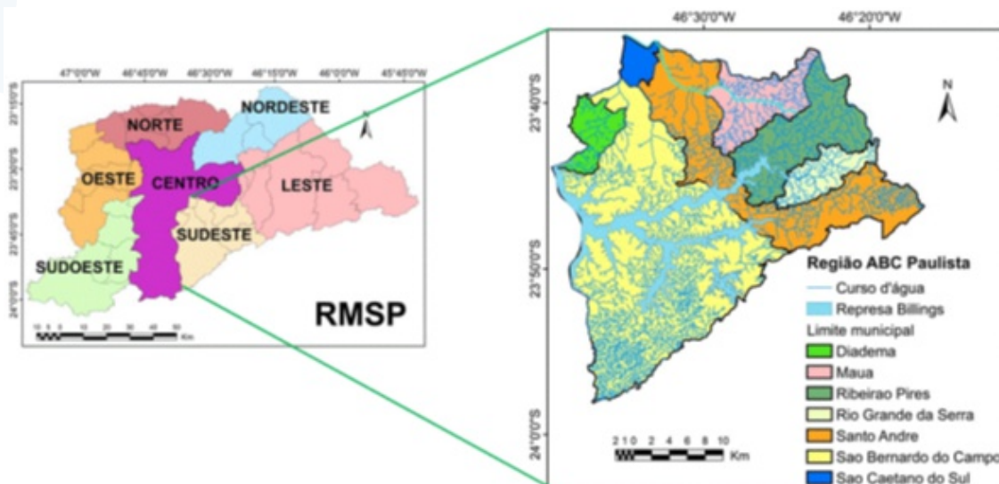
Figura 5 – Mapa da localização da Região do ABC Paulista na Região Metropolitana de São Paulo (RMSP), e sua rede hidrográfica Tamanduateí- Billings
