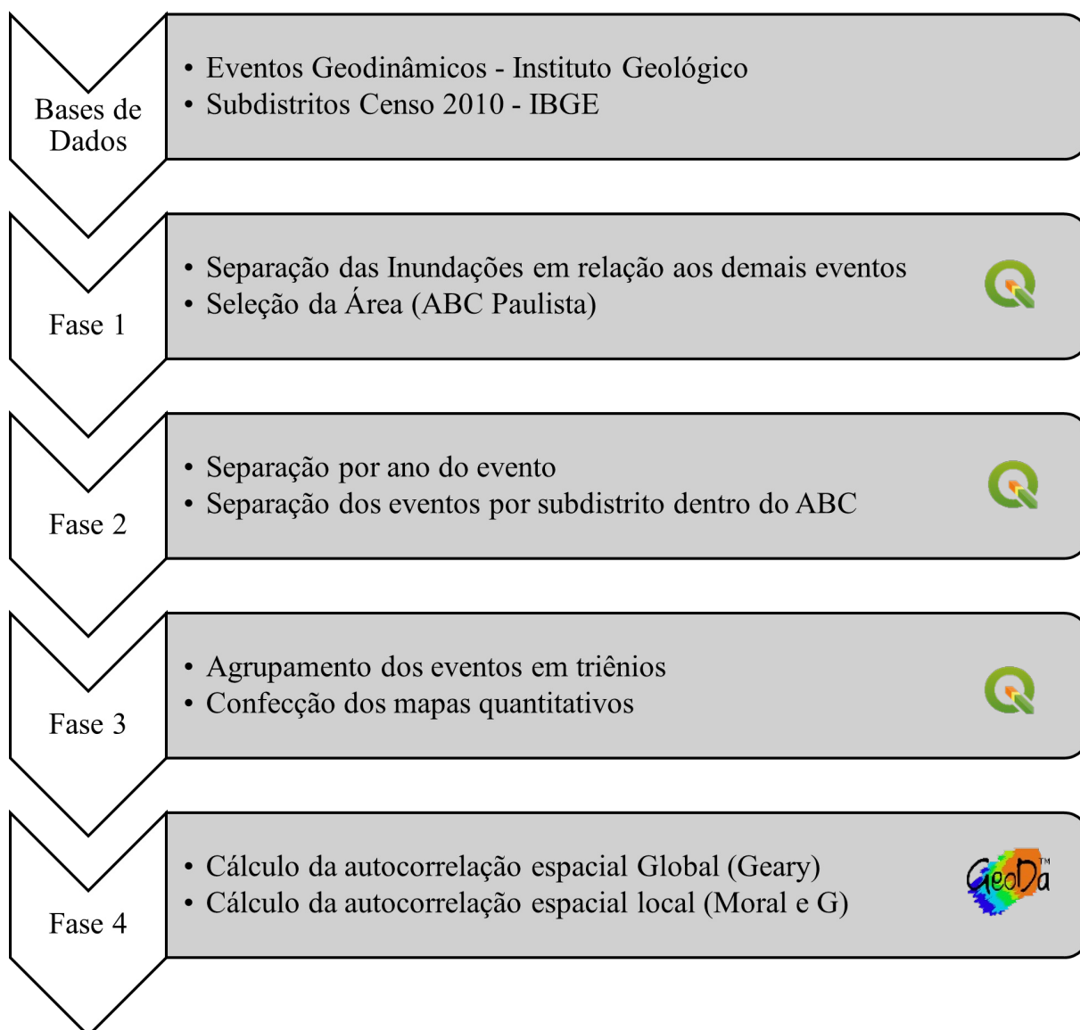
Fluxograma 1: passos do trabalho
