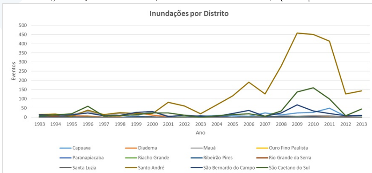
Figura 9 – Quantidade de inundações no ABC Paulista 1993 e 2013, separadas por ano.
