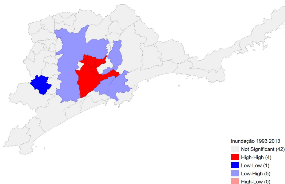
Figura 4 – Teste de autocorrelação de inundações por município na região Metropolitana de SP, Baixada Santista e Litoral Norte entre 1993 e 2013 de acordo com o Índice Local de Moran
